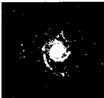
NGC 488
